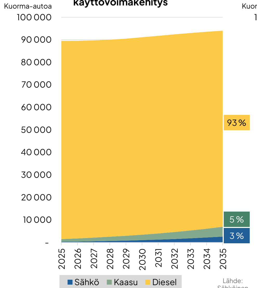
Business as usual- ja bioskenaariot, kuorma-autokannan käyttövoimakehitys
